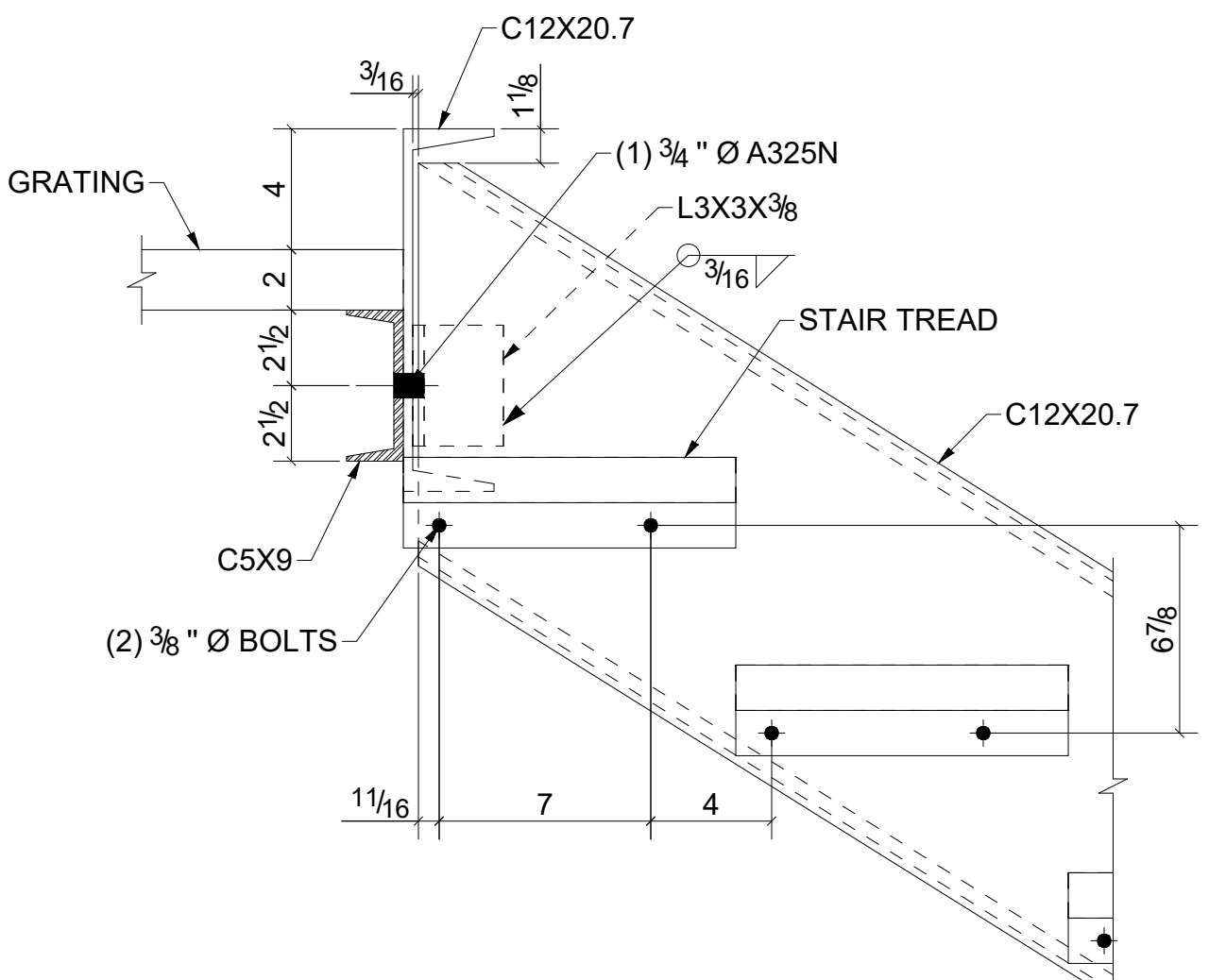
F - F SCALE: 2" = 1'-0"
