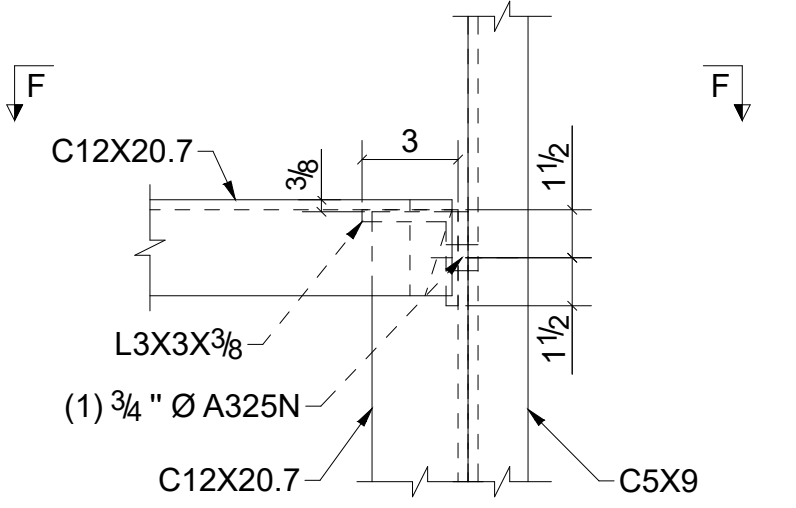
DETAIL 4 SCALE: 2" = 1'-0"
