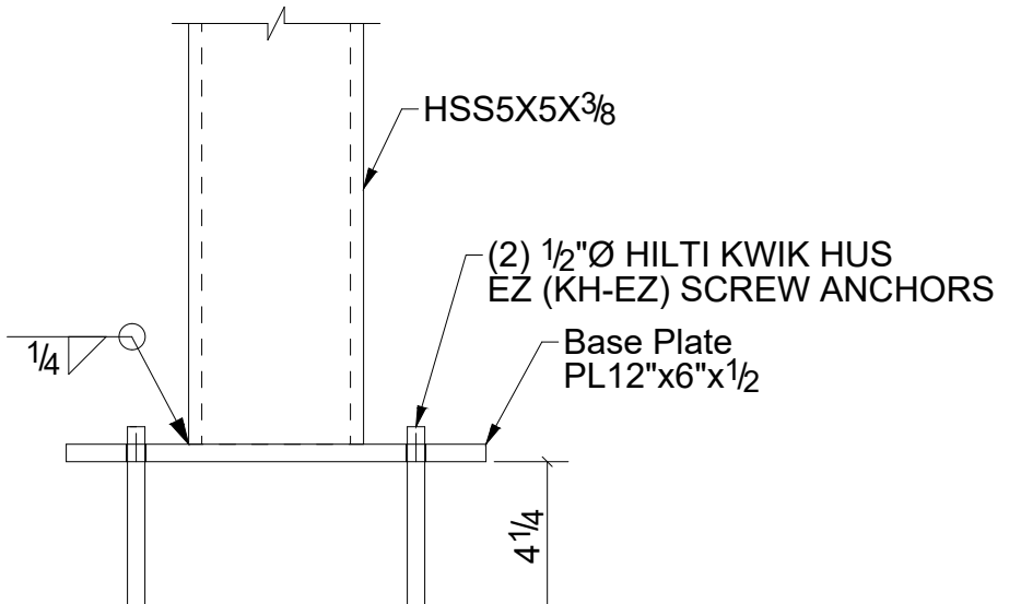
C - C SCALE: 2" = 1'-0"
