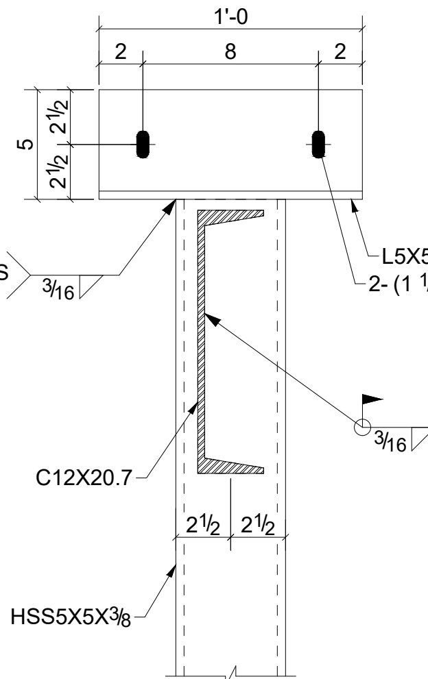
E - E SCALE: 2" = 1'-0"
