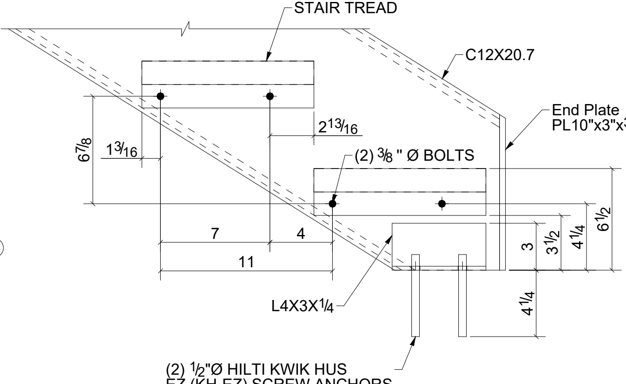
B - B SCALE: 2" = 1'-0"
