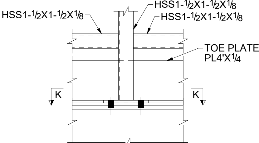
DETAIL 6 SCALE: 2" = 1'-0"
