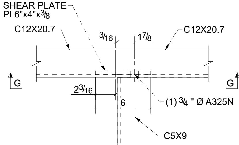
DETAIL 5 SCALE: 2" = 1'-0"
