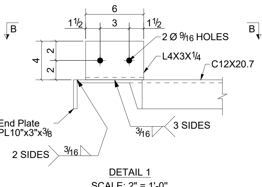
DETAIL 1 SCALE: 2" = 1'-0"
