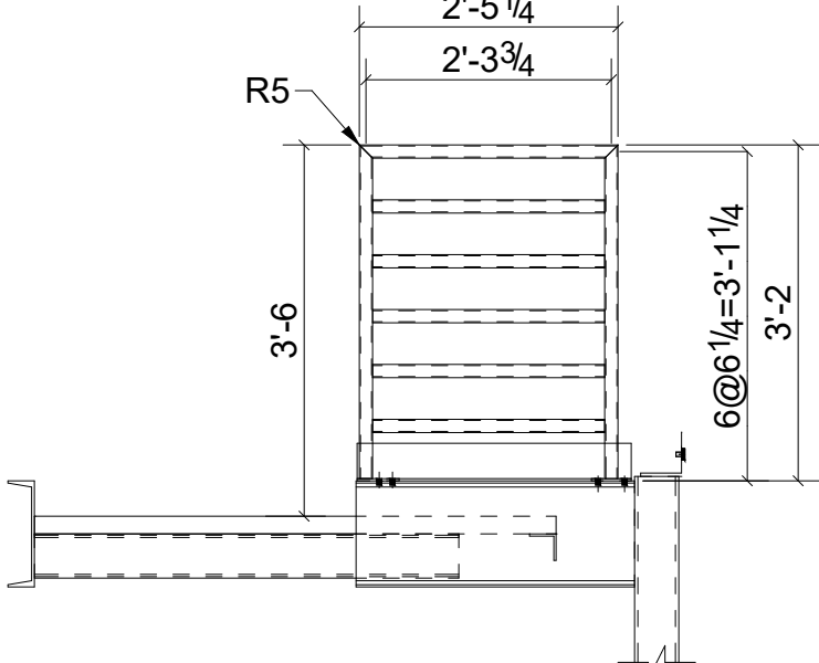
J - J SCALE: 1/2" = 1'-0"
