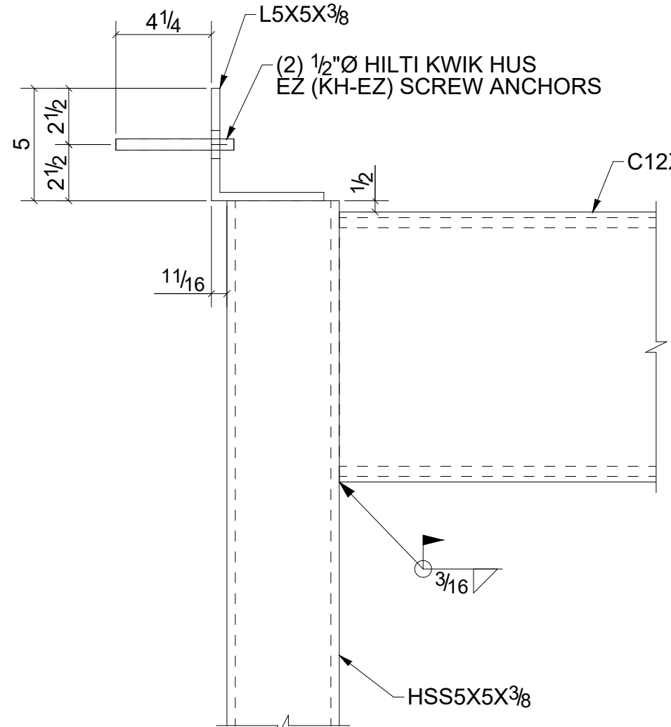
D - D SCALE: 2" = 1'-0"
