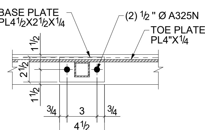
K - K SCALE: 2" = 1'-0"
